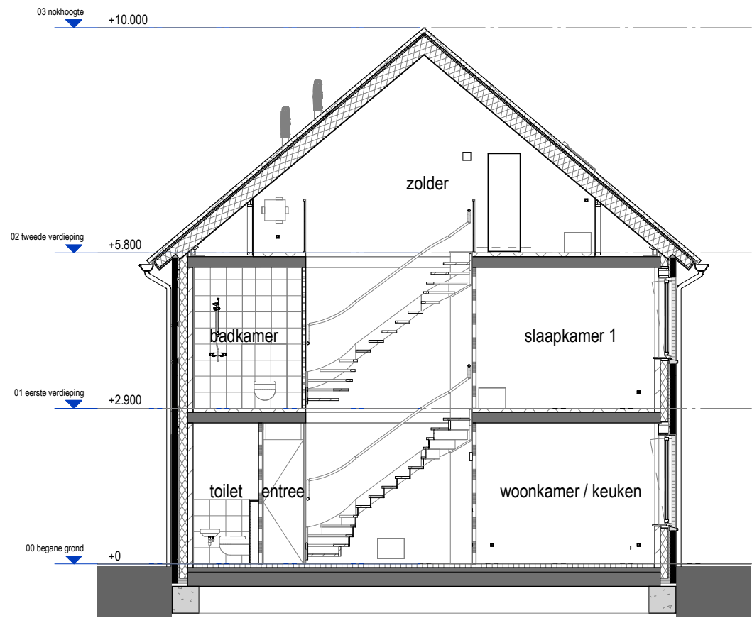
Doorsnede 1 : 100
