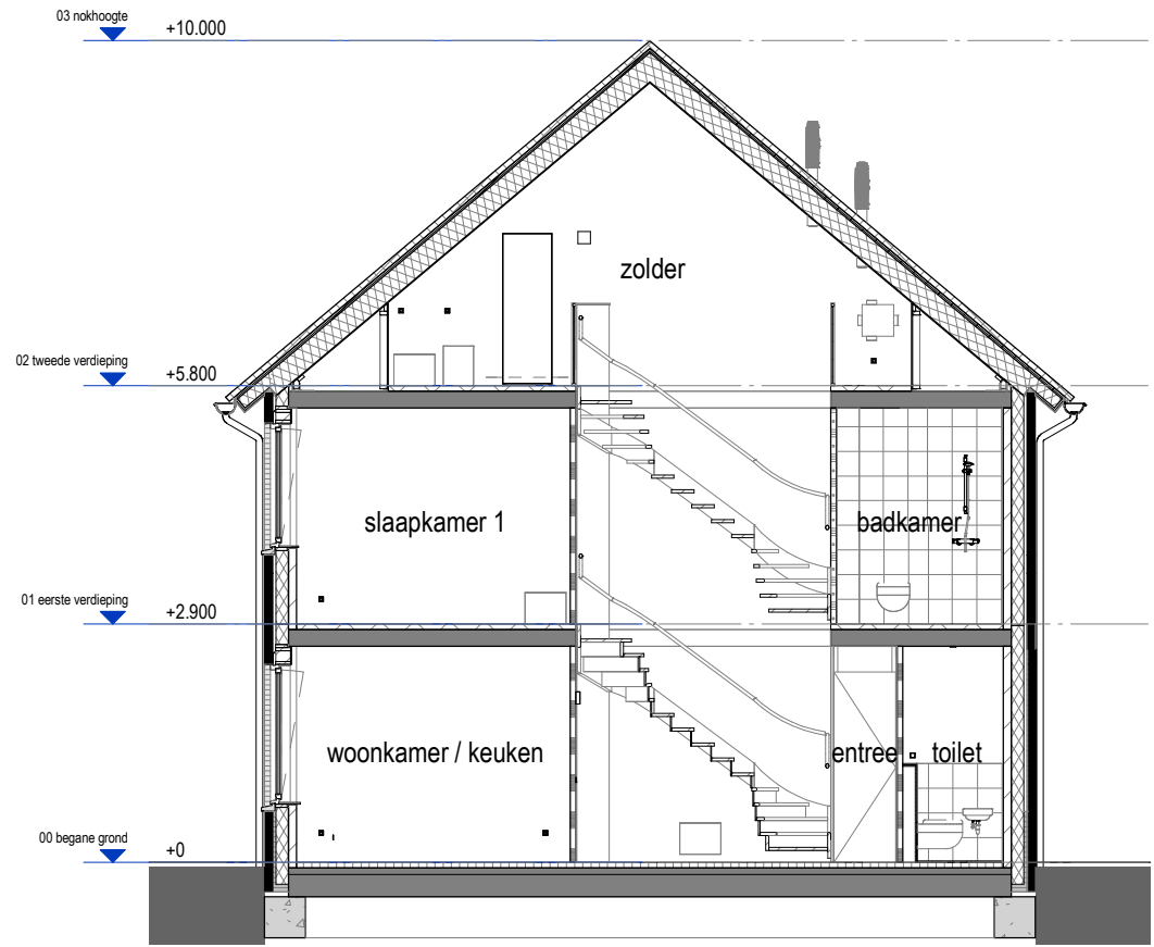
Doorsnede 1 : 100
