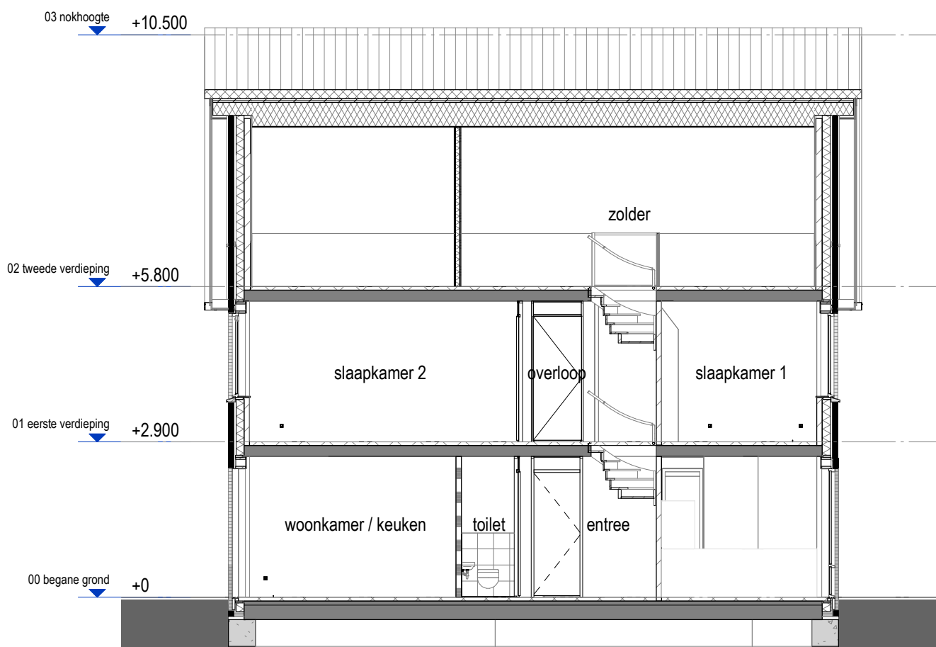
Doorsnede 1 : 100
