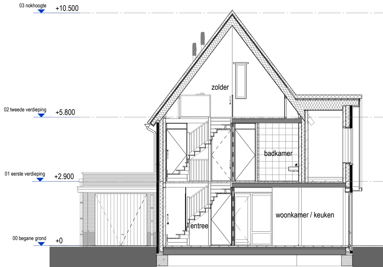
Doorsnede 1 : 100
