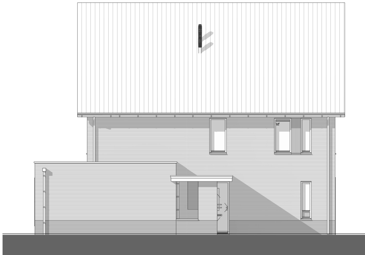
Linker gevel 1 : 100
